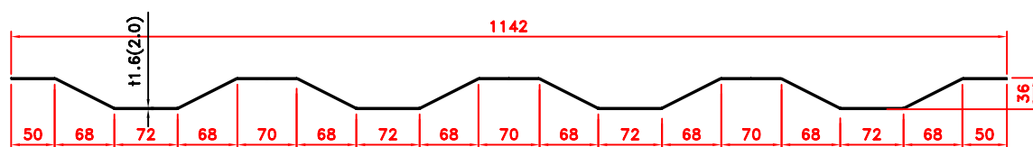
Side Panel 超宽侧板
