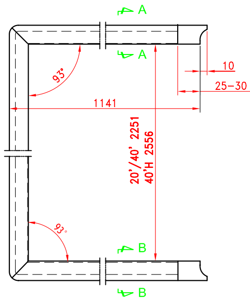
LEFT HAND DOOR ONLY
