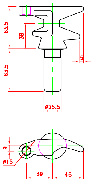
CIMC - D23 - 01C RH (右)
