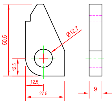
CIMC-D24-06 Hinge Lug SS400
