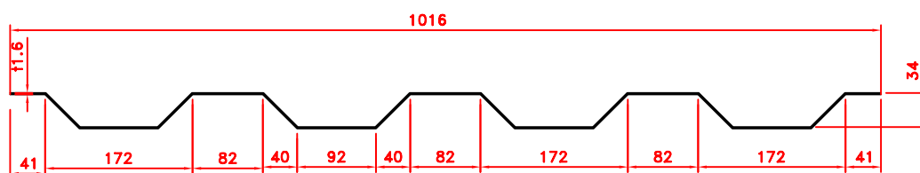
HANJIN Side Panel 韩进侧板
